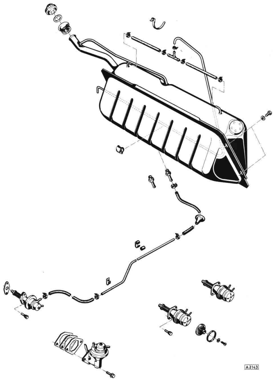
Anordnung Kraftstoffanlage bei Vergaser-Motoren
