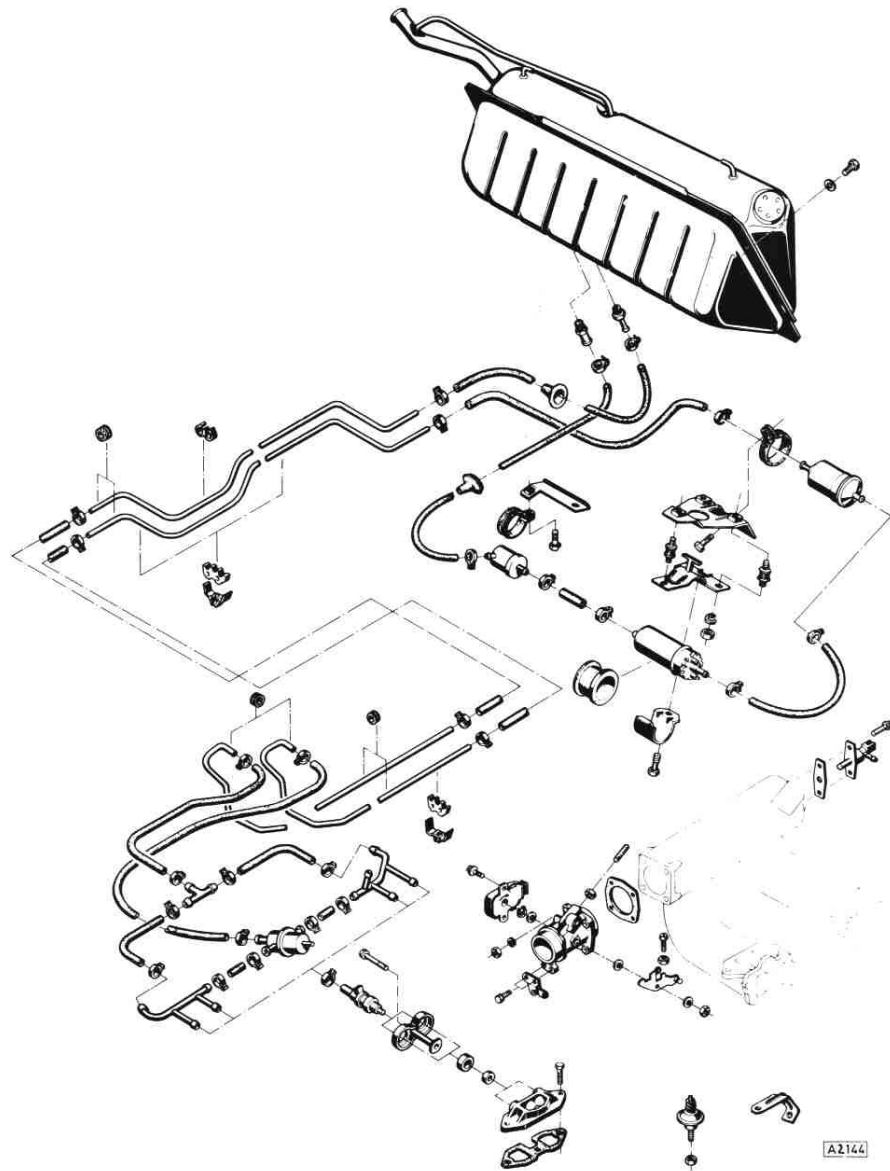
Anordnung Kraftstoffanlage bei E-Motoren
